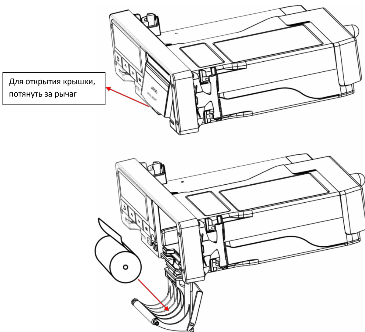
Рисунок 6. Установка бумаги
